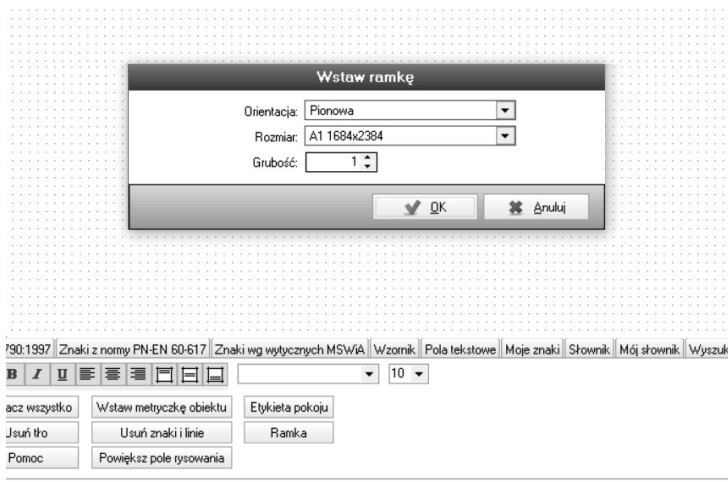
Rys. 5/2.2–4 Dodawanie ramki
