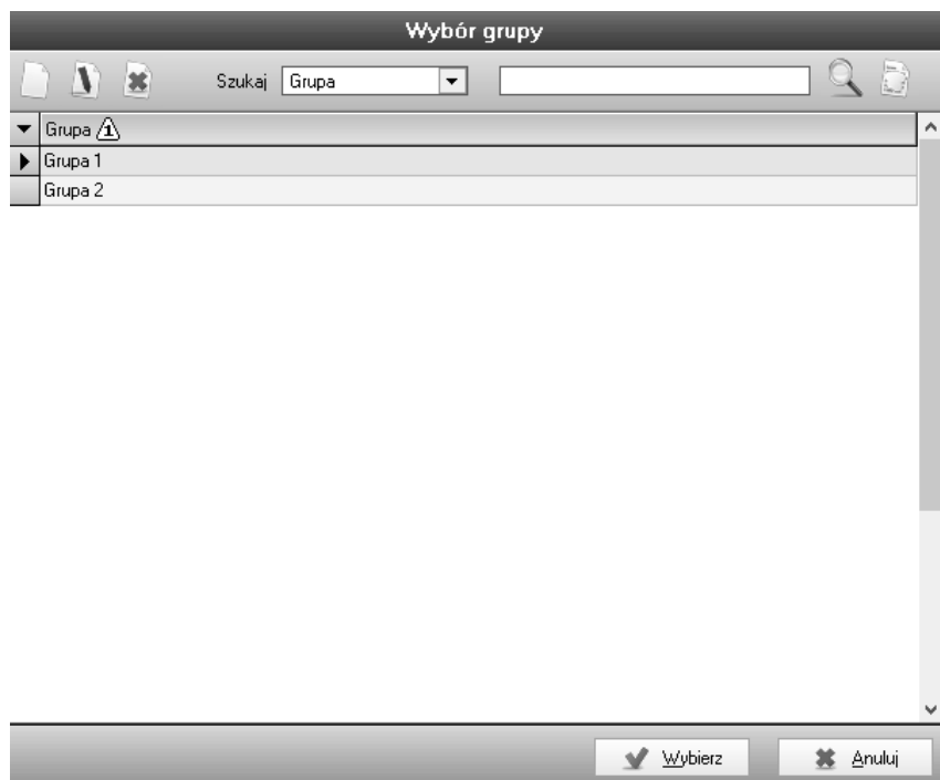
Rys. 5/2.16-2. Wybór grupy
