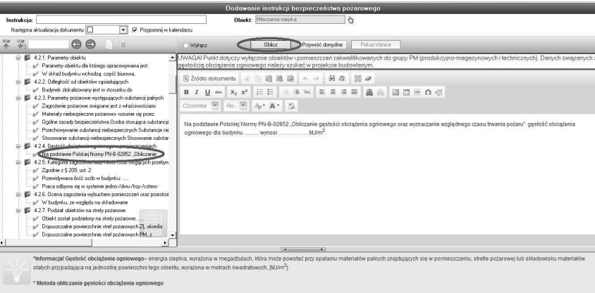
Rys. 5/3.6–1. Przycisk Oblicz
