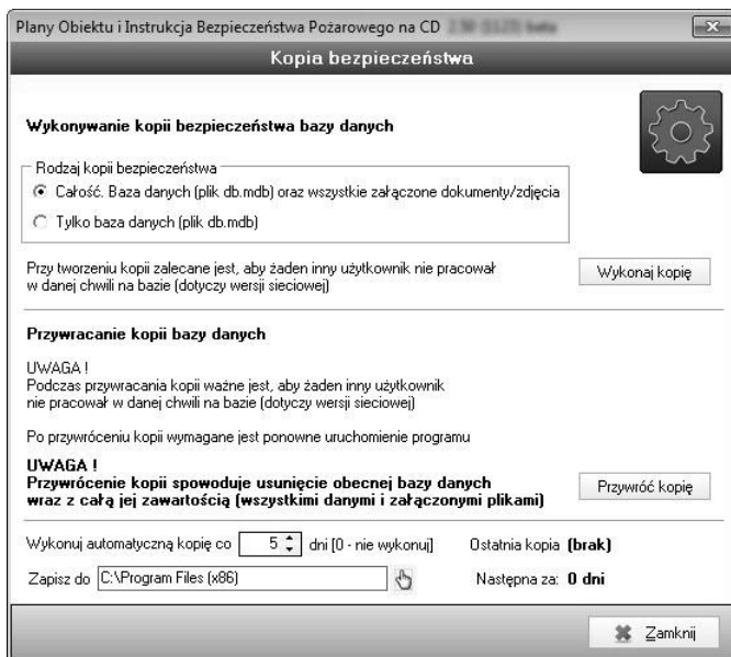
Rys. 2/4–1. Kopia bezpieczeństwa
