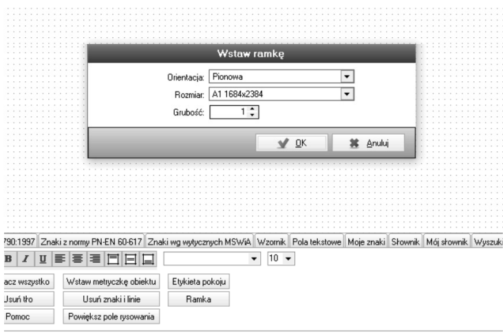
Rys. 5/2.14-1 Dodawanie ramki
