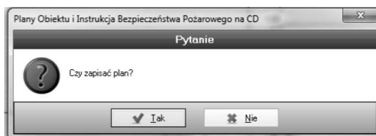
Rys. 4/11.2–2. Okno potwierdzenia
